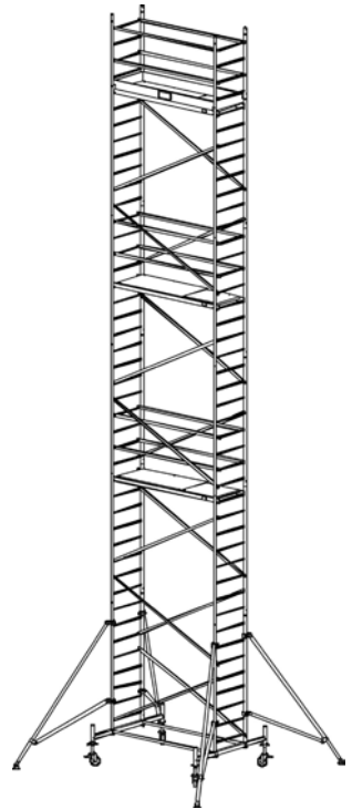
Artikel Nr. Arbeitshöhe: 12,3 m 91 020 2 Gerüsthöhe: 11,3 m Standhöhe: 10,3 m
