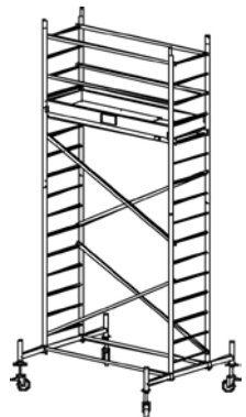
Artikel Nr. Arbeitshöhe: 5,3 m 91 0134 Gerüsthöhe: 4,3 m Standhöhe: 3,3 m
