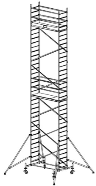
Artikel Nr. Arbeitshöhe: 10,3 m 91 018 9 Gerüsthöhe: 9,3 m Standhöhe: 8,3 m
