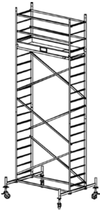
Artikel Nr. Arbeitshöhe: 6,3 m 91 014 1 Gerüsthöhe: 5,3 m Standhöhe: 4,3 m
