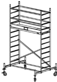
Artikel Nr. Arbeitshöhe: 4,3 m 91 0127 Gerüsthöhe: 3,3 m Standhöhe: 2,3 m
