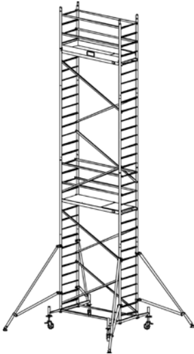
Artikel Nr. Arbeitshöhe: 9,3 m 91 017 2 Gerüsthöhe: 8,3 m Standhöhe: 7,3 m
