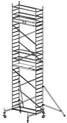
Artikel Nr. Arbeitshöhe: 8,3 m 91 016 5 Gerüsthöhe: 7,3 m Standhöhe: 6,3 m
