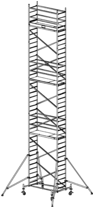
Artikel Nr. Arbeitshöhe: 11,3 m 91 019 6 Gerüsthöhe: 10,3 m Standhöhe: 9,3 m
