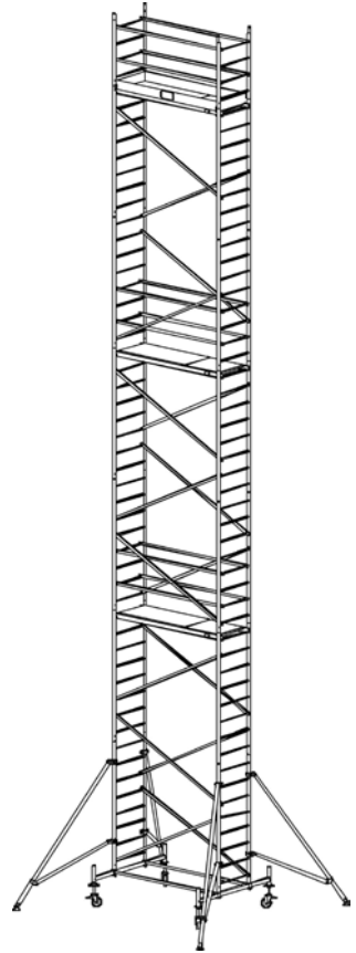
Artikel Nr. Arbeitshöhe: 14,30 m 91 022 6 Gerüsthöhe: 13,3 m Standhöhe: 12,3 m
